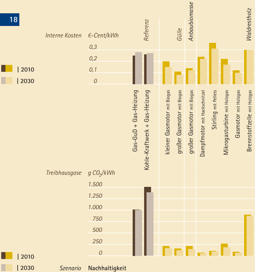
Grafik oben: Kostenbilanz für Strom und Wärme aus Biomasse-KWK im Vergleich zum "Durchschnittsstrom" plus Gasheizung
